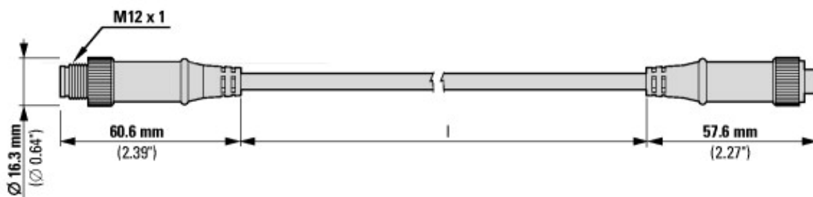
SWD-Rundleitung M12, 5-polig
